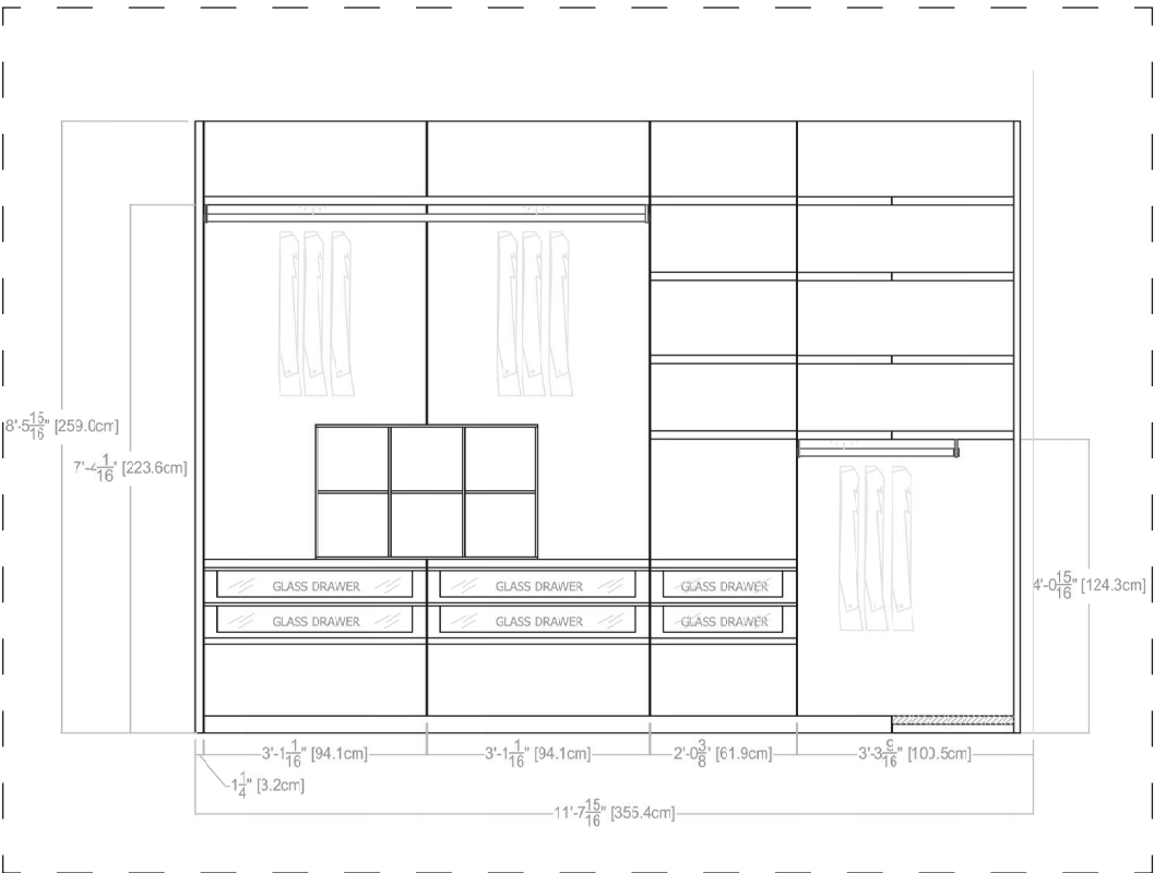
UBIK - ELEVATION A
