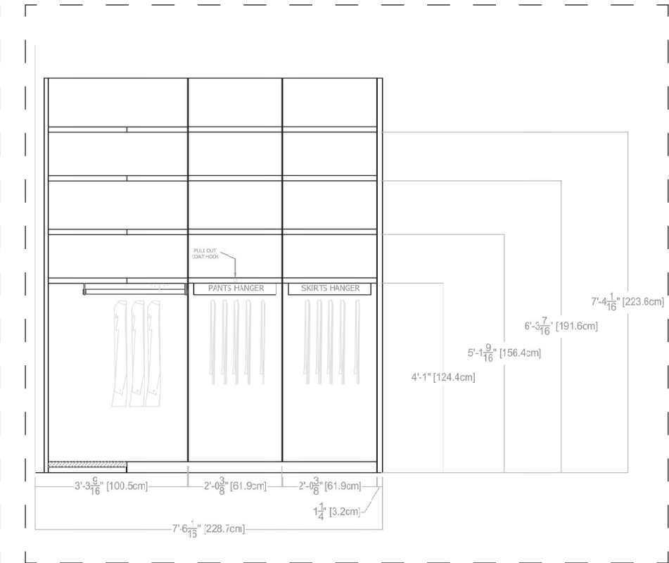
UBIK - ELEVATION B
